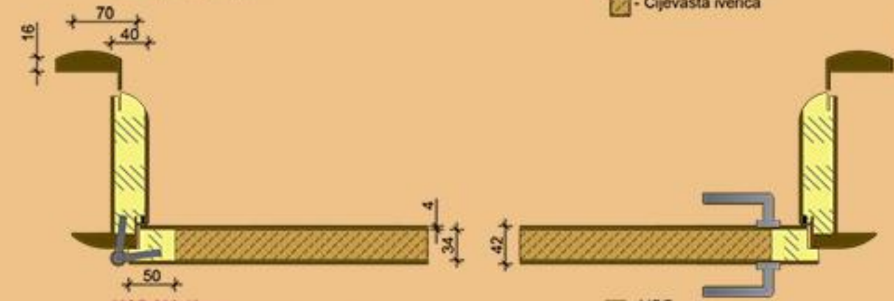
MOD 003 40mm - Oblni dovratnik sa oblim lajsinama - Okov po želji kupca
