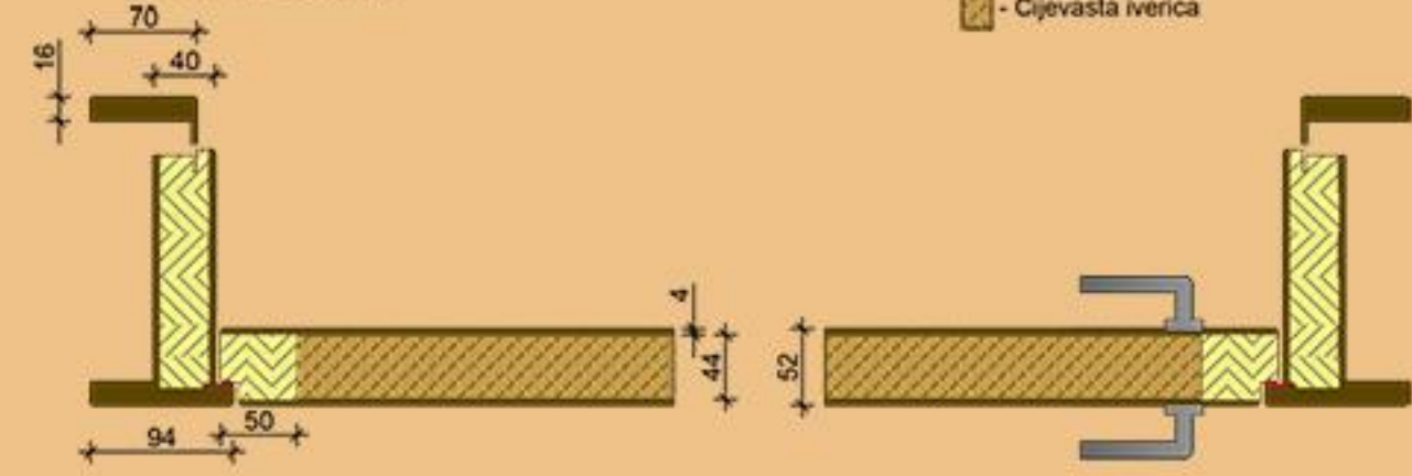
MOD 001 40mm OTVARANJE U DOVRATNIK - Ravni dovratnik sa ravnim lajsinama - Okov po želji kupca
