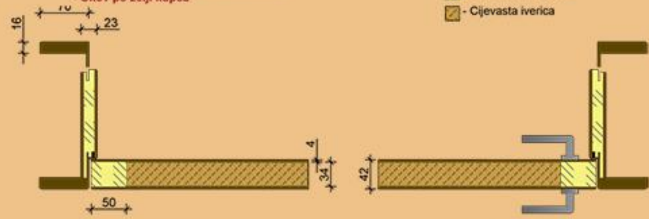
MOD 001 23mm bez falca - Ravni dovratnik sa ravnim lajsinama - Okov po želji kupca
