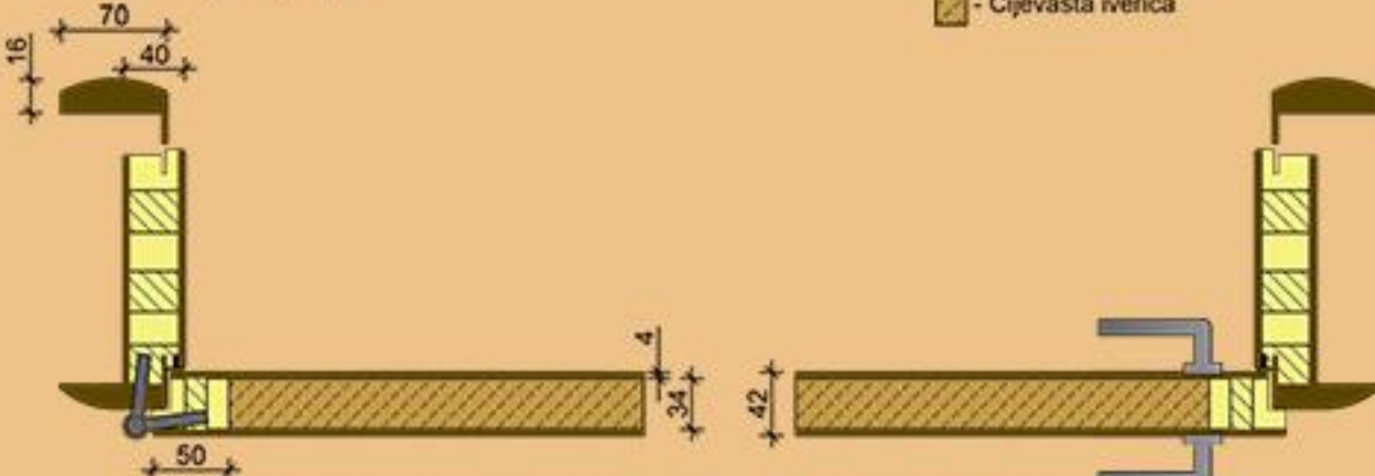
MOD 002 40mm - Ravni dovratnik sa oblim lajsinama - Okov po želji kupca
