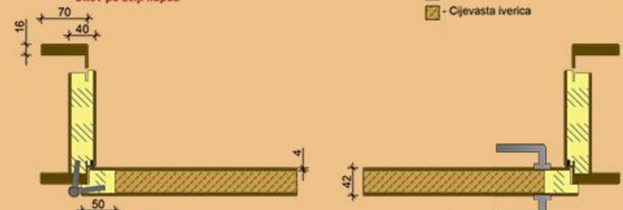
MOD 001 40mm - Ravni dovratnik sa ravnim lajsinama - Okov po želji kupca
