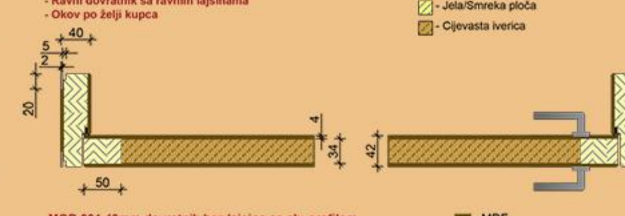
MOD 001 40mm dovratnik bez lajsina sa alu profilom - Ravni dovratnik sa ravnim lajsinama - Okov po želji kupca
