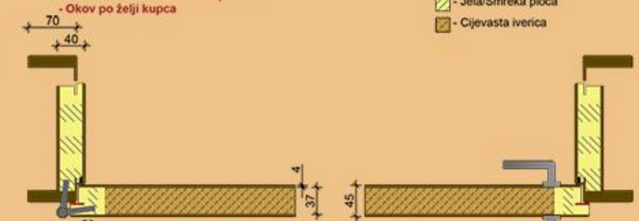
MOD 001 40mm VRATA SA DUPLIM ZAPTIVAČEM - Ravni dovratnik sa ravnim lajsinama - Okov po želji kupca
