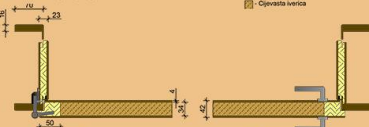
MOD 001 23mm - Ravni dovratnik sa ravnim lajsinama - Okov po želji kupca
