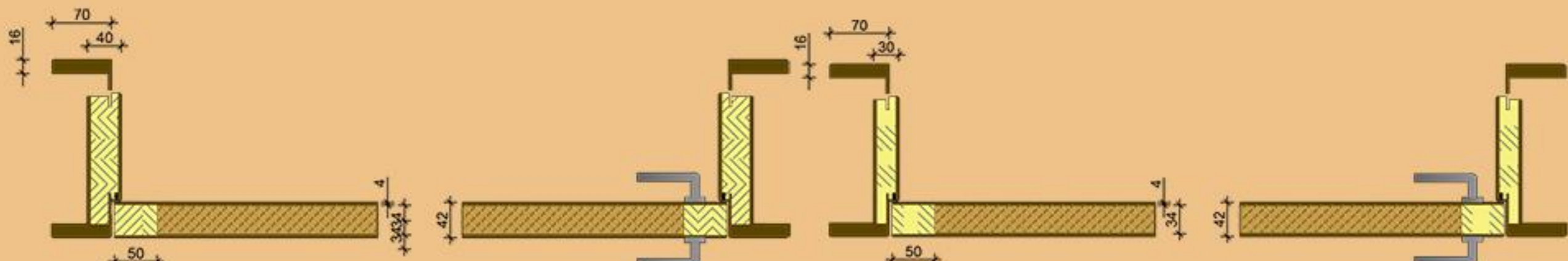
MOD 001 40mm bez falca - Ravni dovratnik sa ravnim lajsinama - Okov po želji kupca
