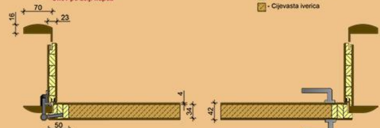
MOD 002 23mm - Ravni dovratnik sa oblim lajsinama - Okov po želji kupca
